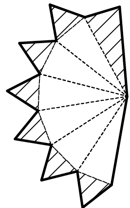
Носовой обтекатель
